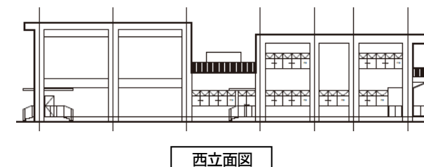
西立面図
