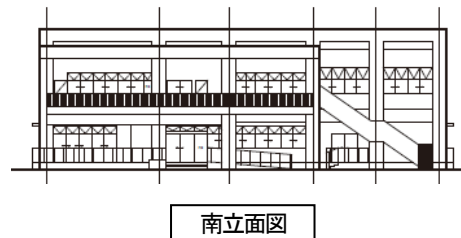
南立面図
