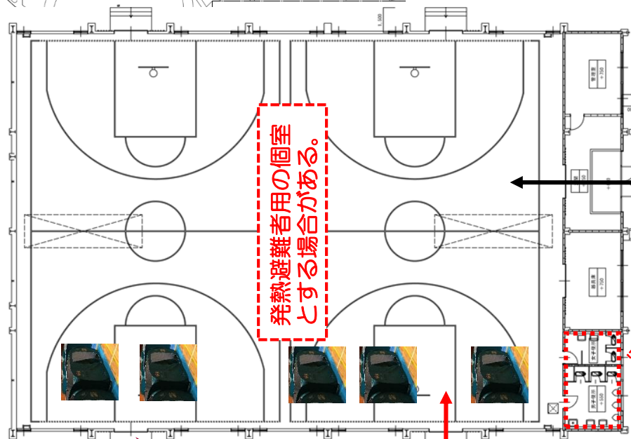
第2 体育館平面図
