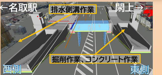
ついに道路横断部の地下道が姿を現し、東西が空間的につながりました。
